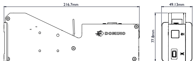
EXT打印头 - 上插口
