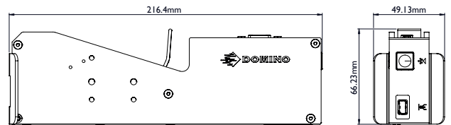
GP打印头 - 上插口
