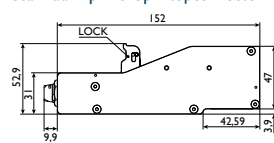
Standaard printkop – topconnector
