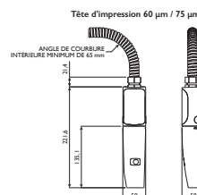
Tête d'impression en acier rond n 60 µm / 75 µm
