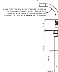
Tête d'impression en acier rond n 60 µm / 75 µm
