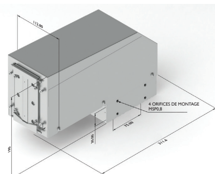
Tête d'impression standard
