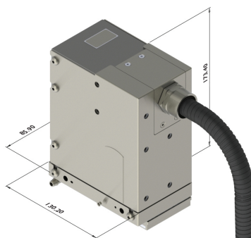
Tête d'impression déportée - verticale
