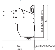
Tête d'impression compacte – Connecteur supérieur
