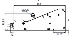
Tête d'impression EXT – Connecteur supérieur
