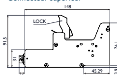
Tête d'impression OPT – Connecteur supérieur
