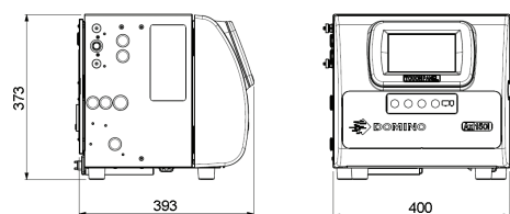
60-µ / 75-µ-Druckkopf
