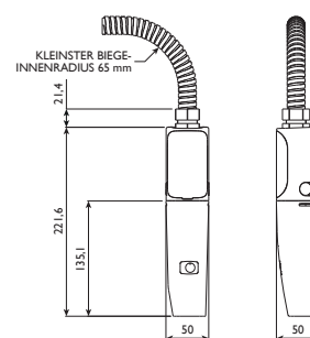
60-µ / 75-µ-Druckkopf
