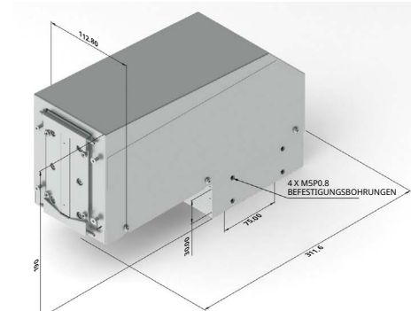
Ausgleichsbehälter dezentraler Druckkopf
