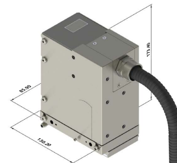
Dezentraler Druckkopf – vertikal
