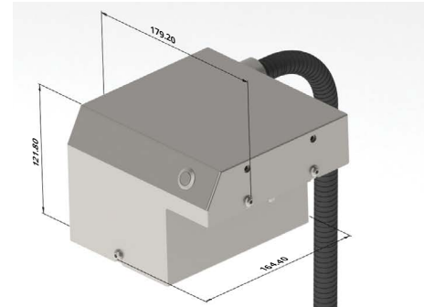
Ausgleichsbehälter dezentraler Druckkopf
