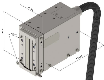
Dezentraler Druckkopf – horizontal
